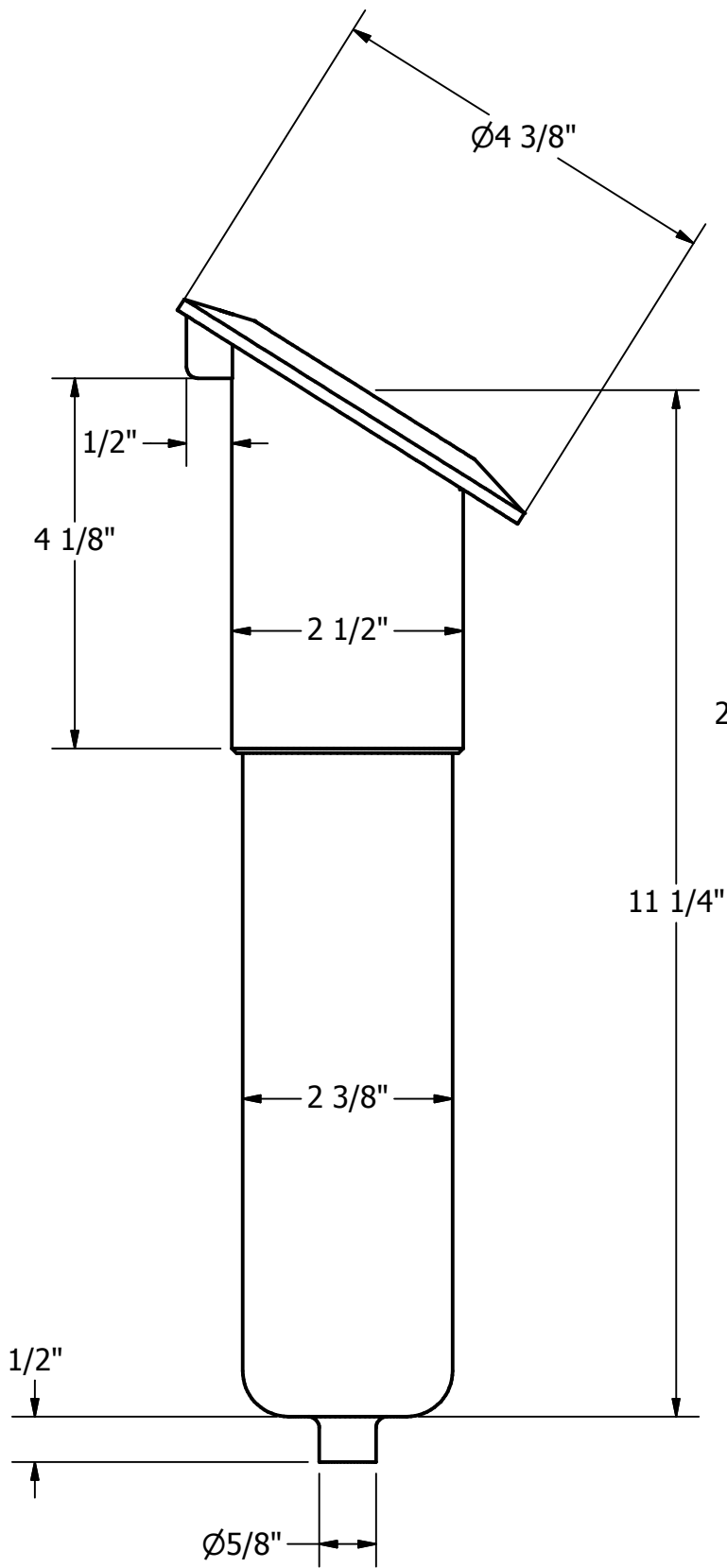
105514 30° HD Rod Holder
