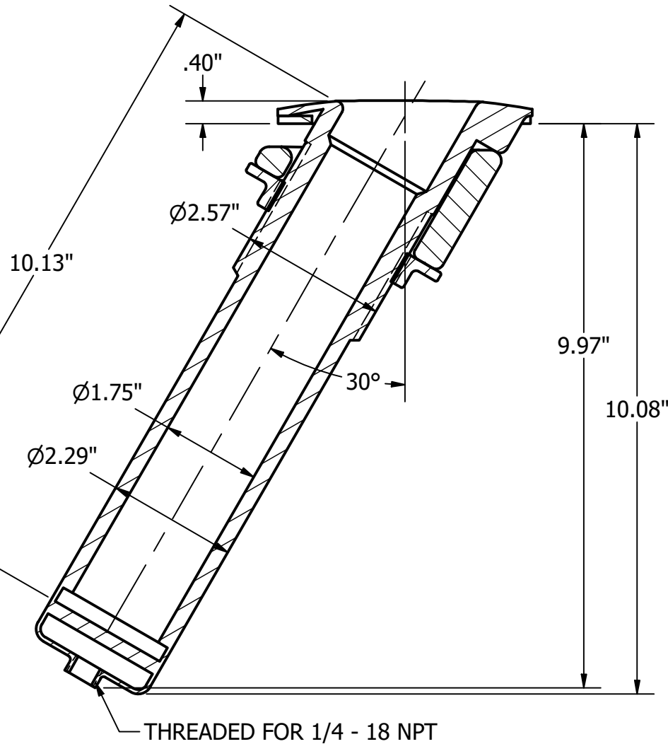
SECTION A-A
