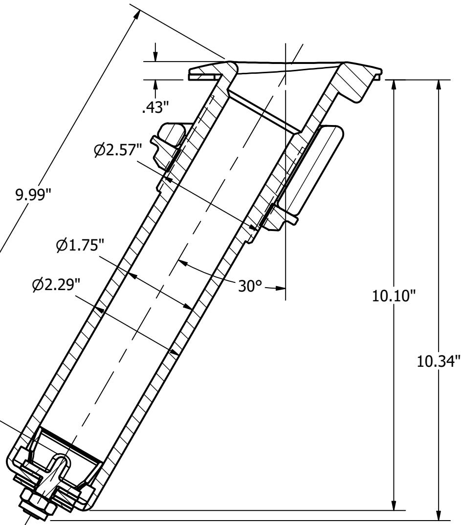
SECTION A-A
